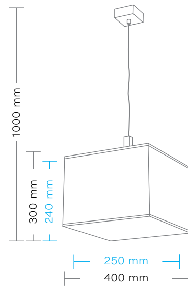
QUATTRO Lampa wisząca/ Hanging lamp max 1 x 40W Gwint/Chip: E27 Zasilanie/Power: 230V
