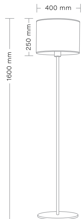
PIANO Lampa stojąca/ Floor lamp max 1 x 40W Gwint/Chip: E27 Zasilanie/Power: 230V
