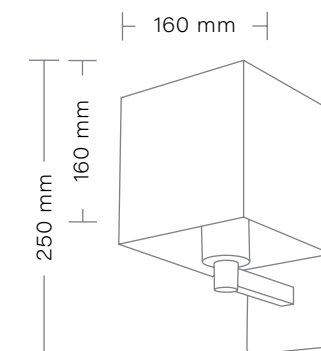
FOBOS Kinkiet/Wall lamp max 1 x 40W Gwint/Chip: E27 Zasilanie/Power: 230V
