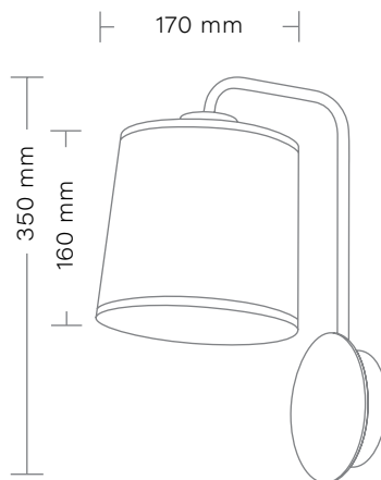
COLUMBUS Kinkiet 3/Wall lamp 3 max 1 x 40W, Gwint/Chip: E27 Zasilanie/Power: 230V
