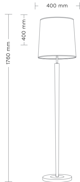
PLATAN Lampa stojąca/ Floor lamp max 1 x 40W Gwint/Chip: E27 Zasilanie/Power: 230V
