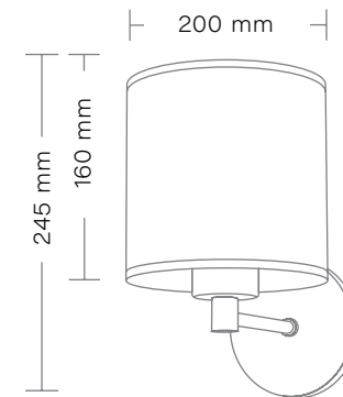
DOS Kinkiet 1/Wall lamp 1 max 1 x 40W Gwint/Chip: E27 Zasilanie/Power: 230V
